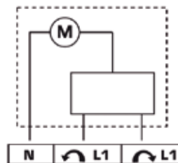
Esquema eléctrico
